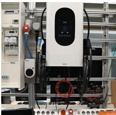
Abbildung 24 | Inbetriebnahme einer bidirektionalen E-Ladesäule.
