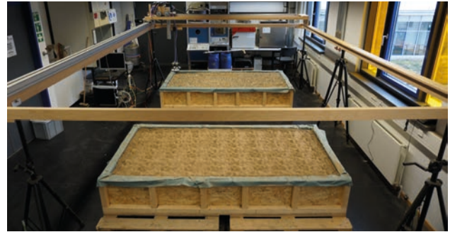
Abbildungen 28/29 | Metalldetektor an einer Drohne zum Aufspüren von Antipersonenminen (links), Bodenmessplatz Find Mine-Projekte (rechts); Quelle: THU
