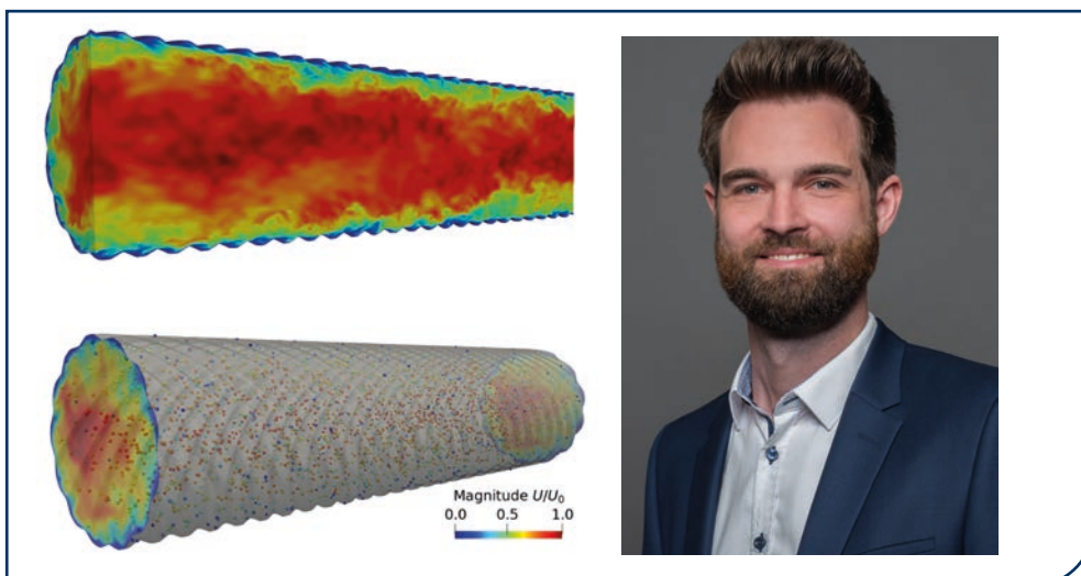
Abbildung 7 | Illustration der turbulenten Rohrströmung und der inneren Partikelposition. RE = 16000 Momentanes Geschwindigkeitsfeld (oben) und Partikelposition (unten). Die Flüssigkeitsbewegung erfolgt von links nach rechts. Quelle: Akermann/THU
