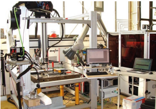
Abbildungen 31/ 32 | Versuchsaufbau zum Heißdraht unterstützten MSG-Auftragschweißen (links), Hochgeschwindigkeitsaufnahme des Heißdraht unterstützten MSG-Prozesses (rechts); Quelle: THU
