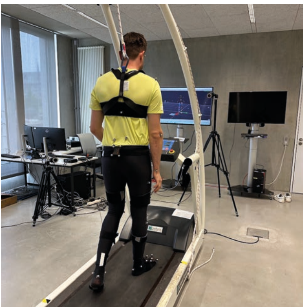
Abbildung 20 | Gang-Messung eines Probanden mit Kamera-System und Inertialsensoren zur Generierung von Trainingsdaten für das KI-System im Bewegungsanalyse-Labor der Forschungsgruppe Biomechatronik
