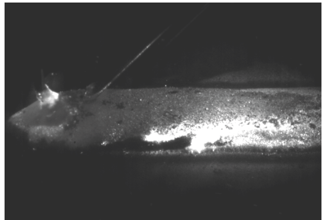
Abbildungen 31/ 32 | Versuchsaufbau zum Heißdraht unterstützten MSG-Auftragschweißen (links), Hochgeschwindigkeitsaufnahme des Heißdraht unterstützten MSG-Prozesses (rechts); Quelle: THU
