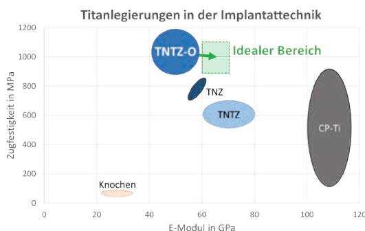
Abbildung 33 | Einordnung der mechanischen Eigenschaften von TNTZ-O unter den Titanlegierungen für Implantatanwendungen; Quelle: THU
