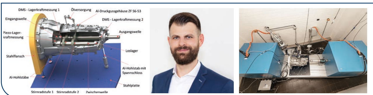
Abbildung 10 | Erweiterter Getriebeprüfstand, Quelle: Werner/THU
