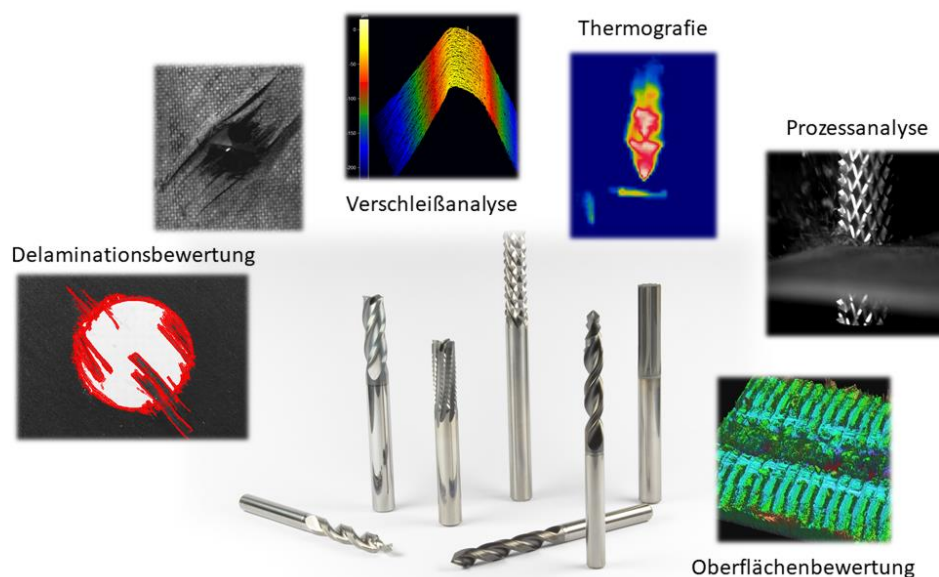
Bild 2: Einblick in die Analysemethoden für das Werkzeugbenchmarking.
